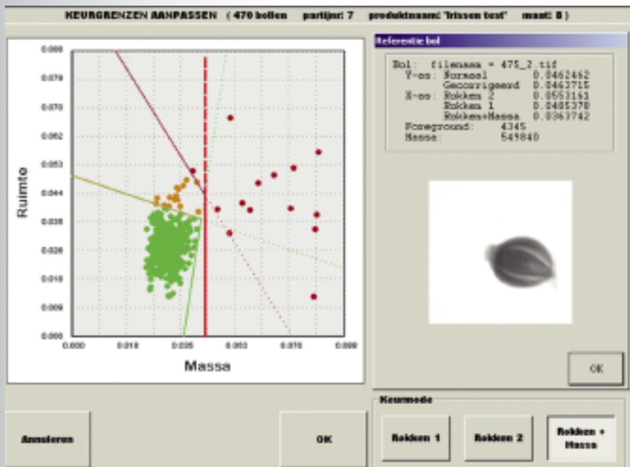
Figuur 3: Eenvoudig instellen van de machine via een touchscreen.
